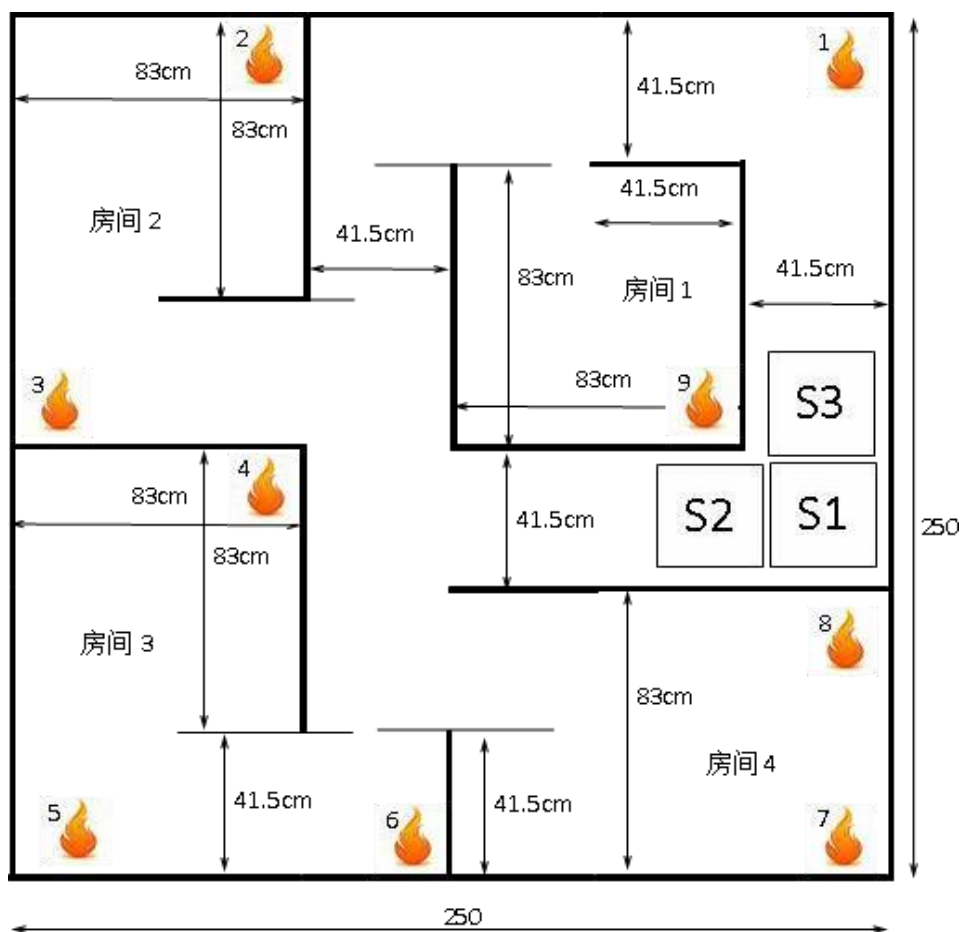
图 1 灭火场地
